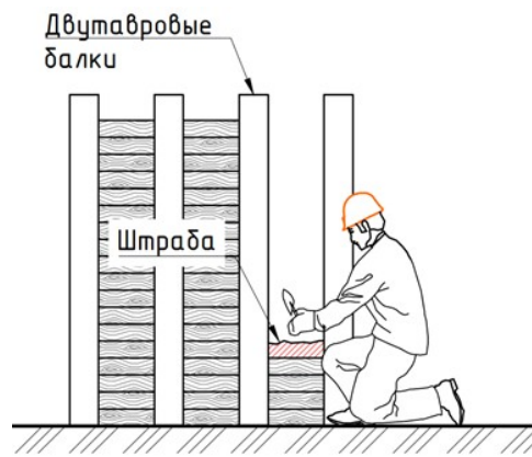
Схема устройства штрабы
