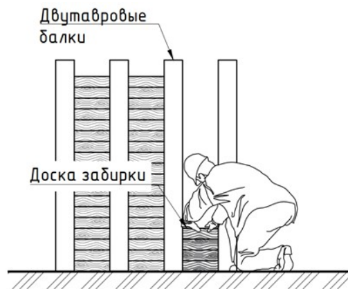
Схема установки досок
