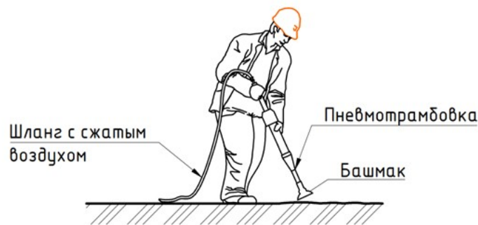
Схема уплотнения грунта пневматическими трамбовками
