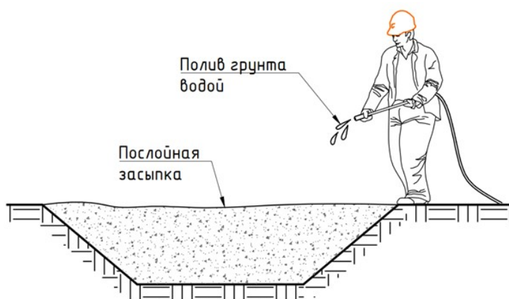
Схема полива грунта водой
