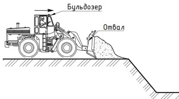
Схема засыпки выемки
