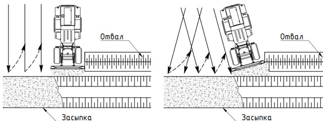
Схема засыпки бульдозером перпендикулярными и косыми проходами
