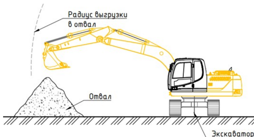
Схема погрузки грунта в отвал
