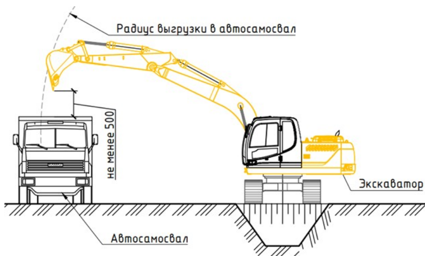
Схема погрузки грунта на автомобили-самосвалы
