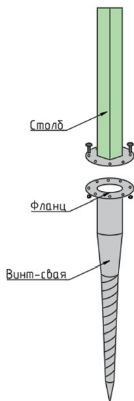
Схема варианта монтажа столба ограждения на винт-сваю (Сечения показаны условно)
