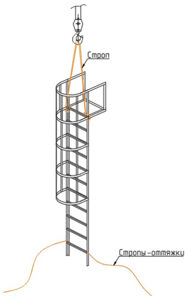
Схемы строповки секций пожарных лестниц (Сечение конструкции показано условно)
