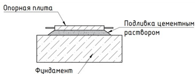
Схема подливки опорной плиты (Элементы крепления условно не показаны)
