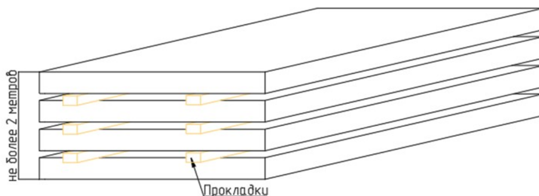
Схема складирования плит лоджий Плиты лоджии показана условно
