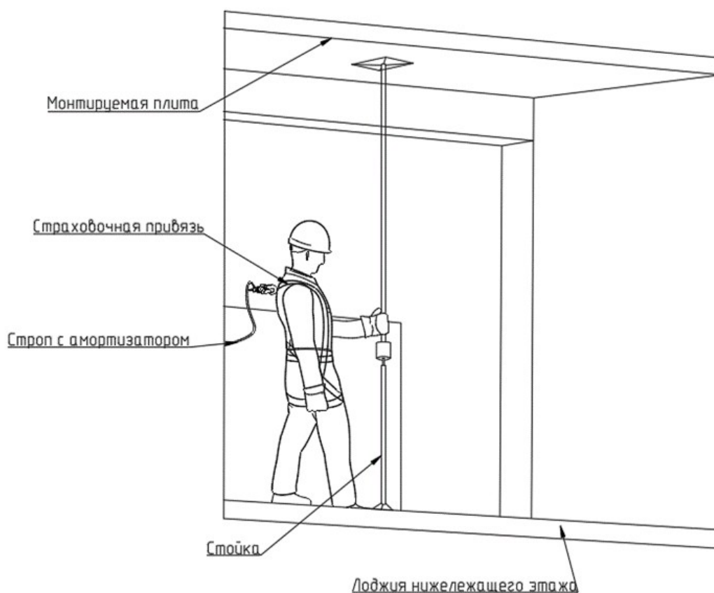
Схема производства работ
