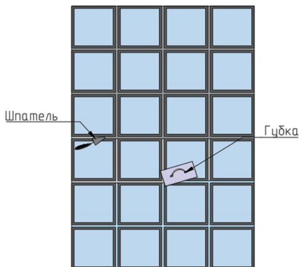
Схема оформления стыков
