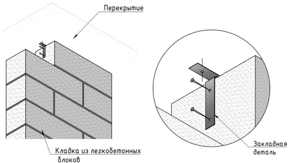
Схема крепления кладки к перекрытию (Вид снизу)
