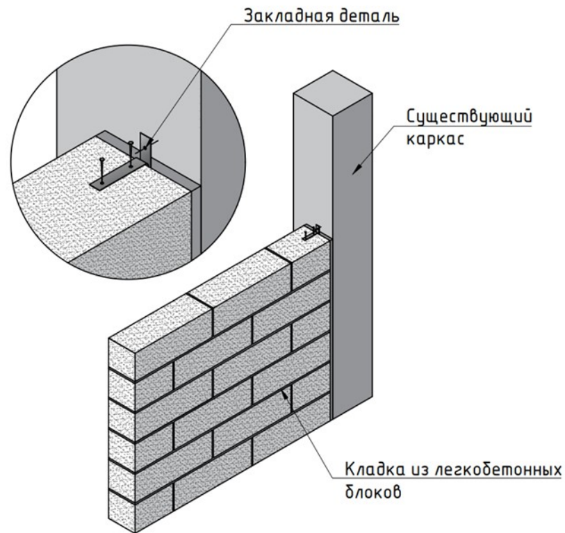
Схема крепления кладки в каркасу
