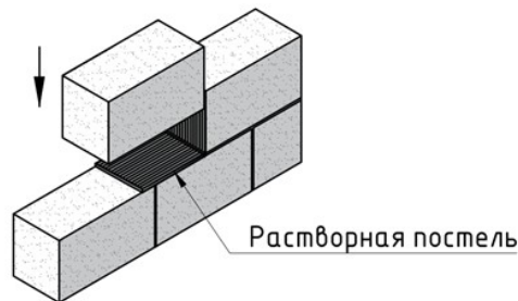
Схема укладки легкобетонного камня
