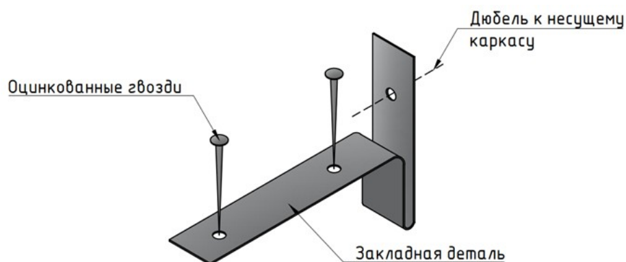
Схема устройства закладной детали
