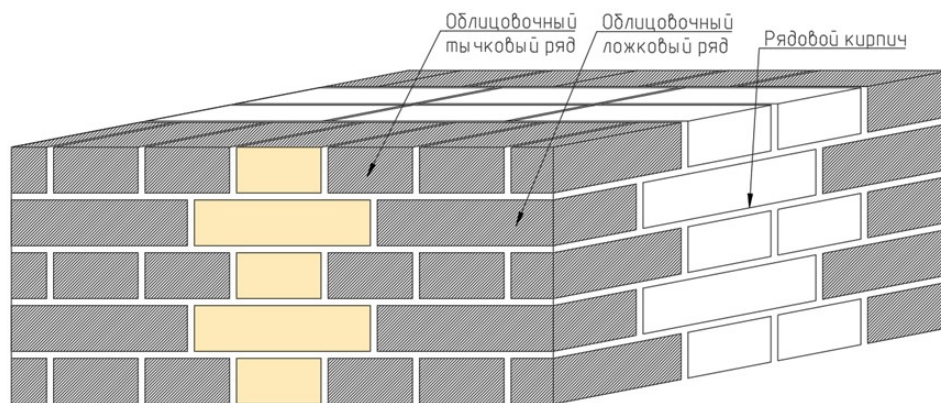
Схема облицовки цепной кирпичной кладки (Желтым цветом обозначена схема цепной перевязки кладки)
