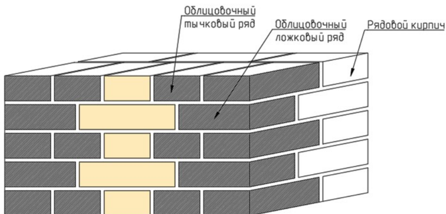
Схема облицовки цепной кирпичной кладки (Желтым цветом обозначена схема цепной перевязки кладки)
