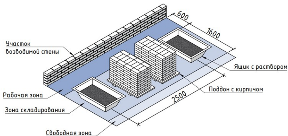
Схема организации рабочего места каменщика
