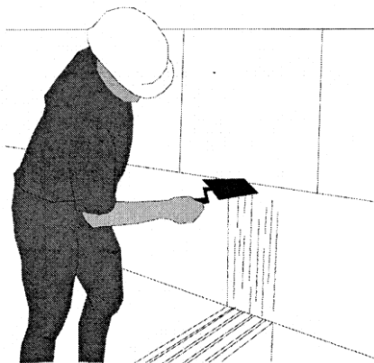
Рисунок 40 – Нанесение раствора для тонкошовной кладки на возведенную стену - нанести раствор для тонкошовной кладки на примыкающий к возведенной стене элемент кладки (рисунок 41);
