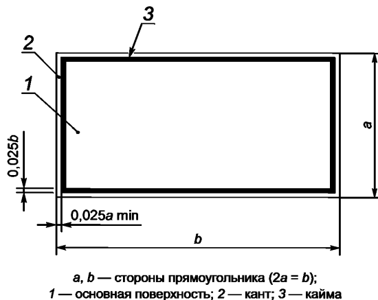
Рисунок 7 — Основа цветографического изображения и соотношение размеров дополнительных знаков безопасности
