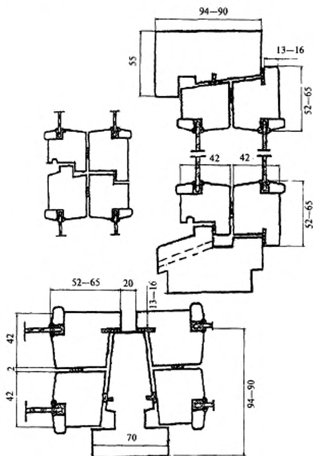
Рисунок 3 – Примеры конструктивных решений оконных блоков спаренной конструкции (с распашным открыванием створок, двумя рядами уплотняющих прокладок, наплав толщиной 16 мм – под ввертнутую петлю)
