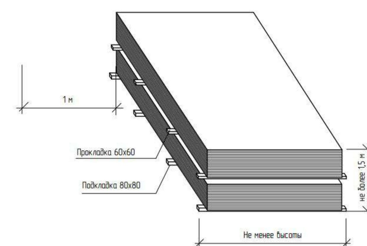
Порядок складирования листовых материалов в стеллажах
