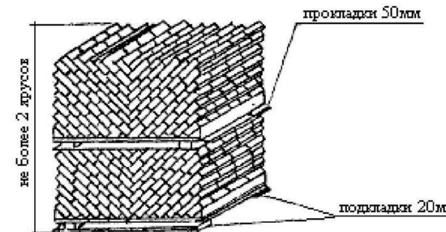
Схема складирования кирпича и пугилобской плитки
