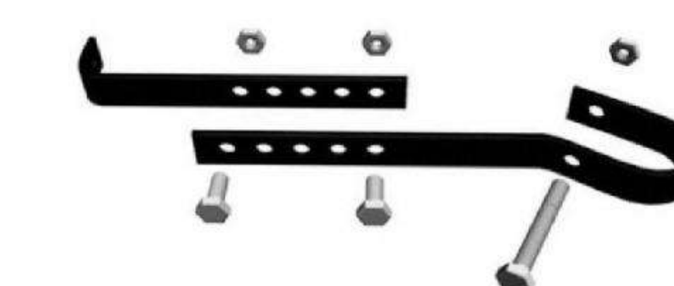
Кронштейн для крепления лесов к стене
