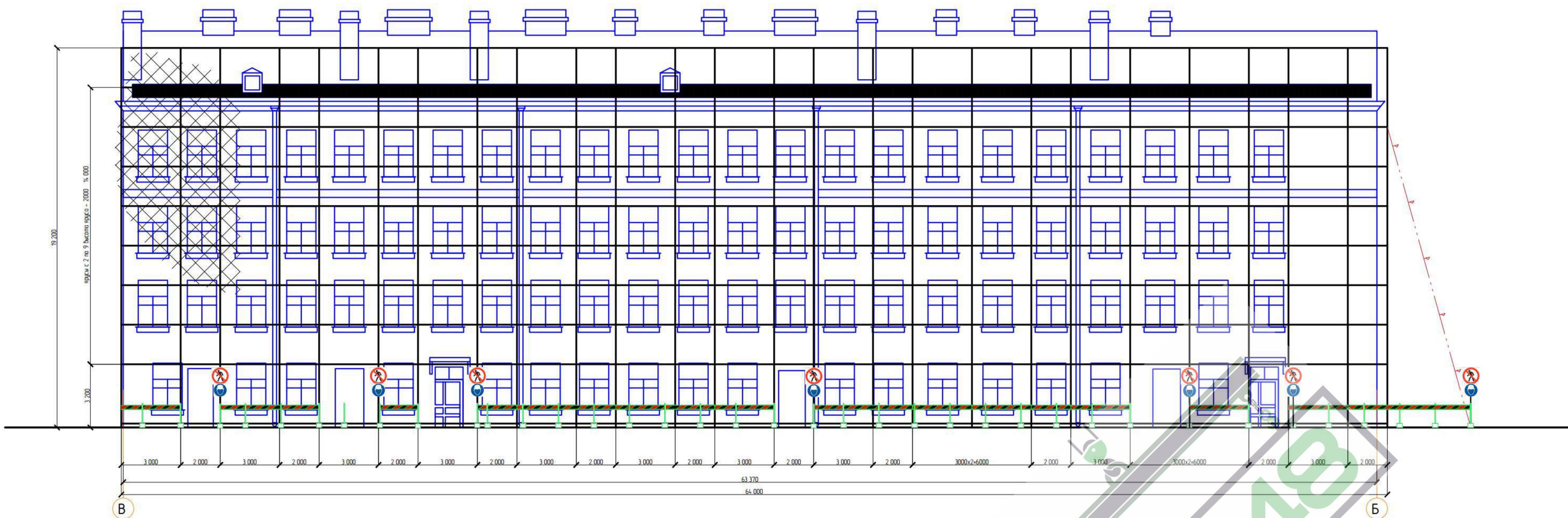
Схема расстановки лесов на фасаде Б-Д
