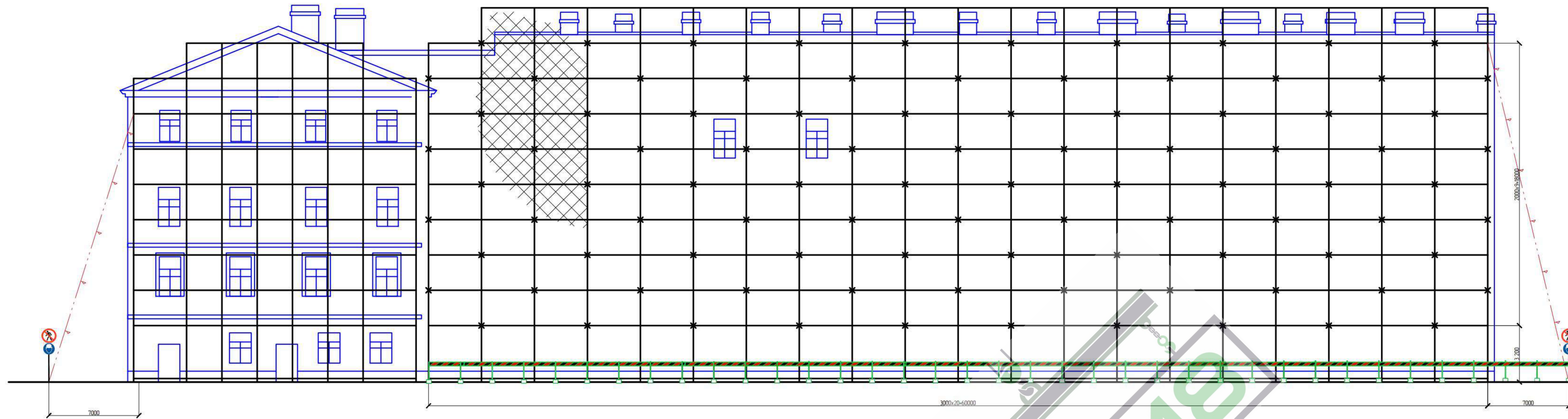
Схема крепления лесов к стене
