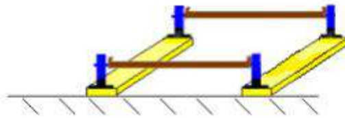
— Рис. 6 – 4 этап: в стартовые элементы вставить вертикальные стойки строго по уровню.
