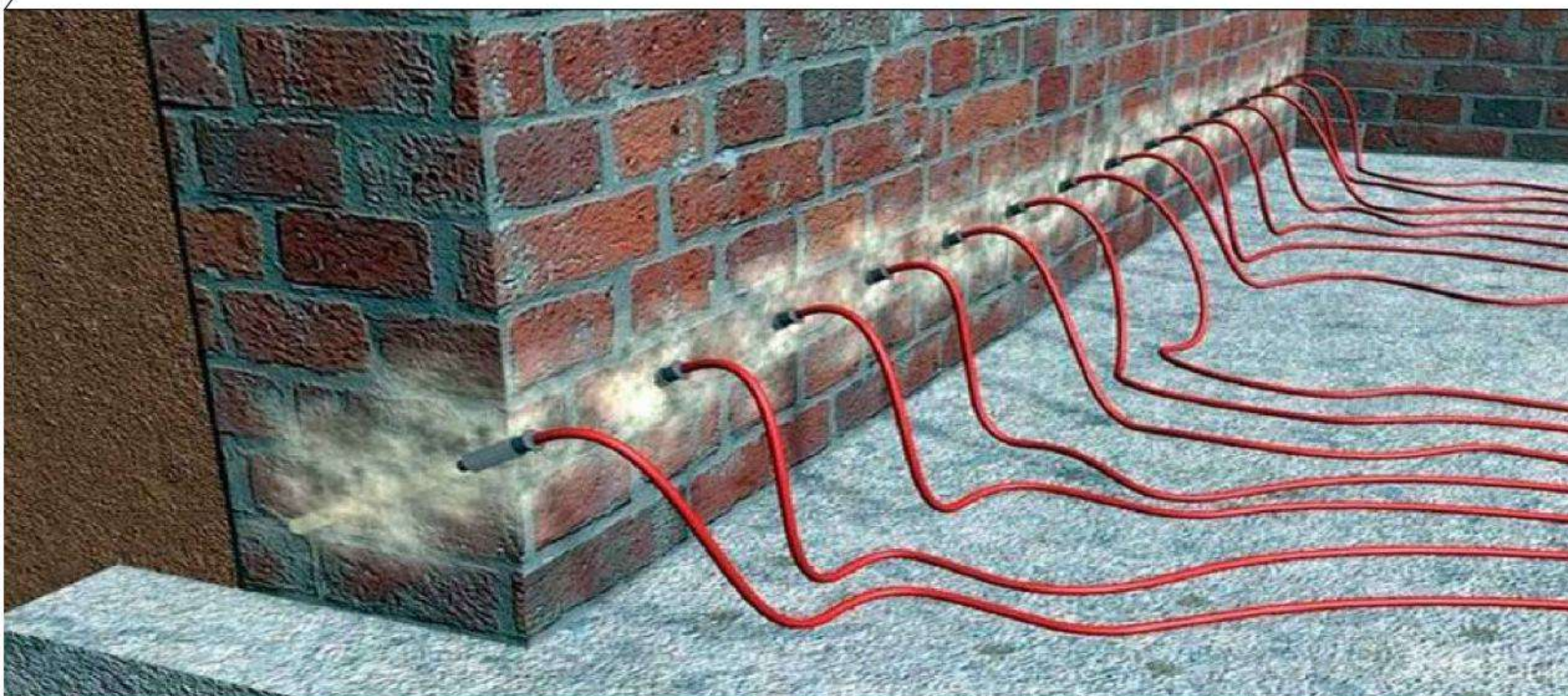
Схема инъектирования состава КАЛЬМАТРОН
