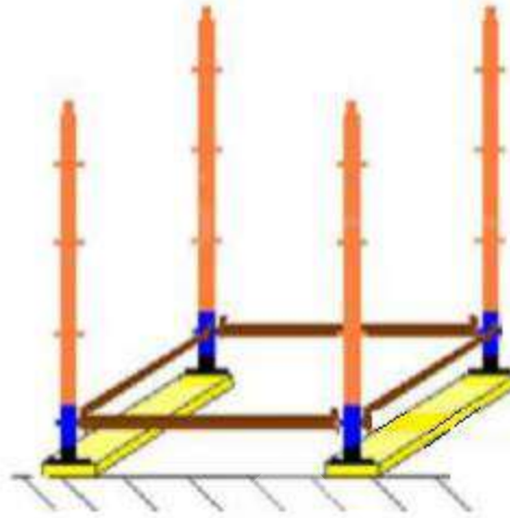
— Рис. 7 – 5 этап: на уровне 0,4; 2,4 метра и т.п. установить горизонтальные связи, соблюдая при этом угол между продольными и поперечными элементами строго 90^\circ . После монтажа горизонтальных связей закрепить вертикальные стойки к стене с помощью кронштейнов.
