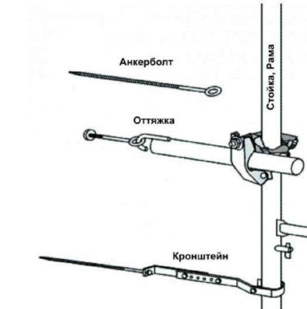
Схема крепления лесов к стене
