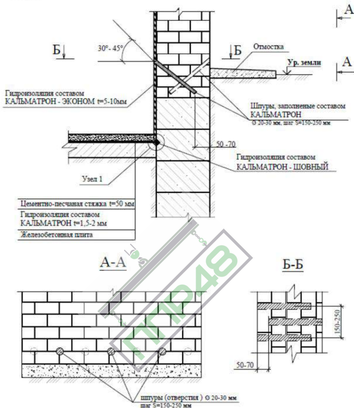
Рис. 17 Пример устройства шпуров в конструкции под инъектирование гидроизоляционным составом. По настоящему ППР предполагается инъектирование конструкции фундамента в обозначенных проектом местах
